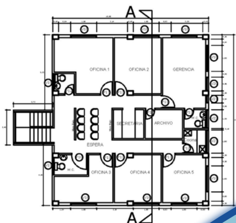
PLANTA SEGUNDO PISO PROYECTO
